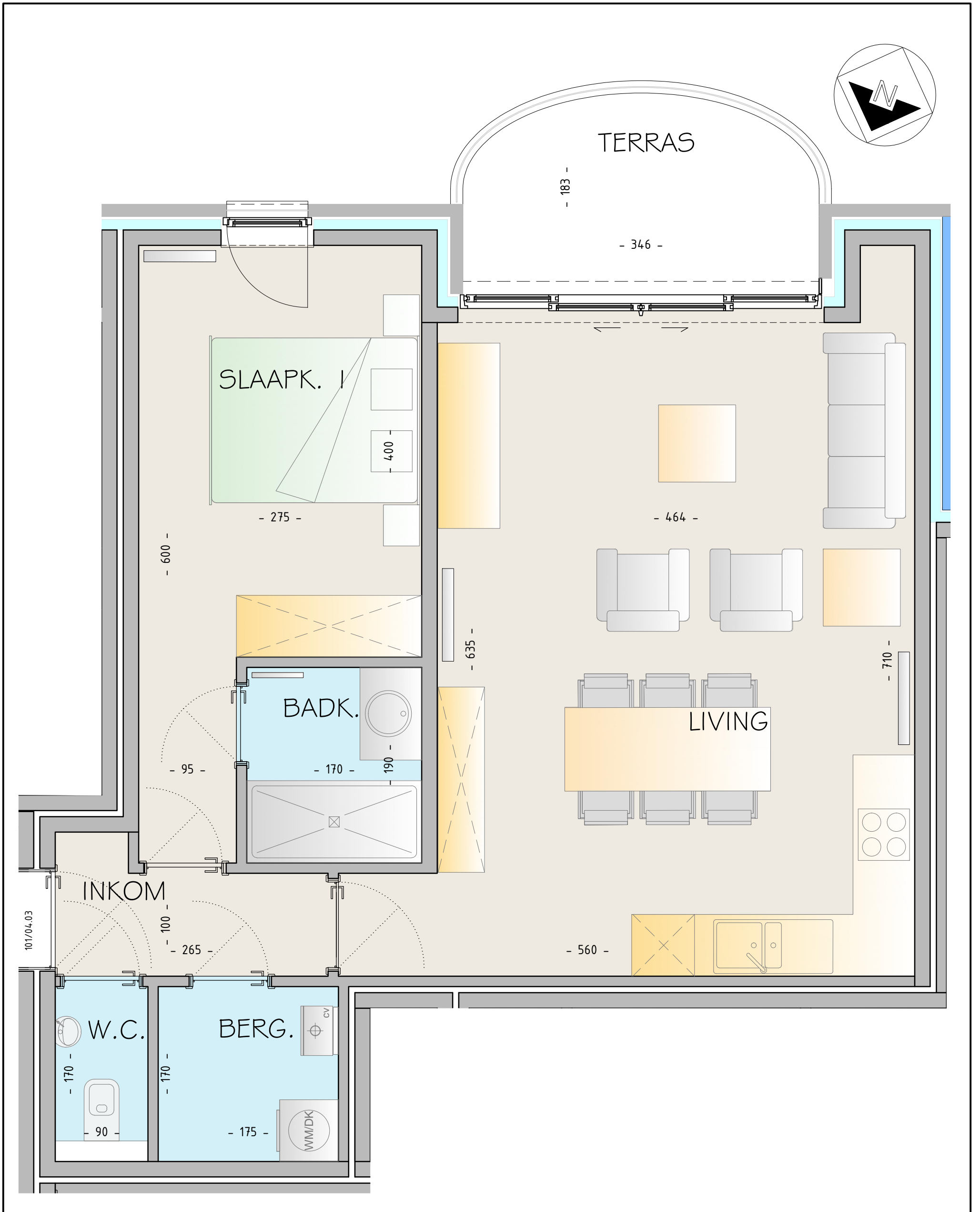
Appartement 101 / 05.03 Koninklijke Baan - B-8670 KOKSIJDE plandatum: 01/03/2019
