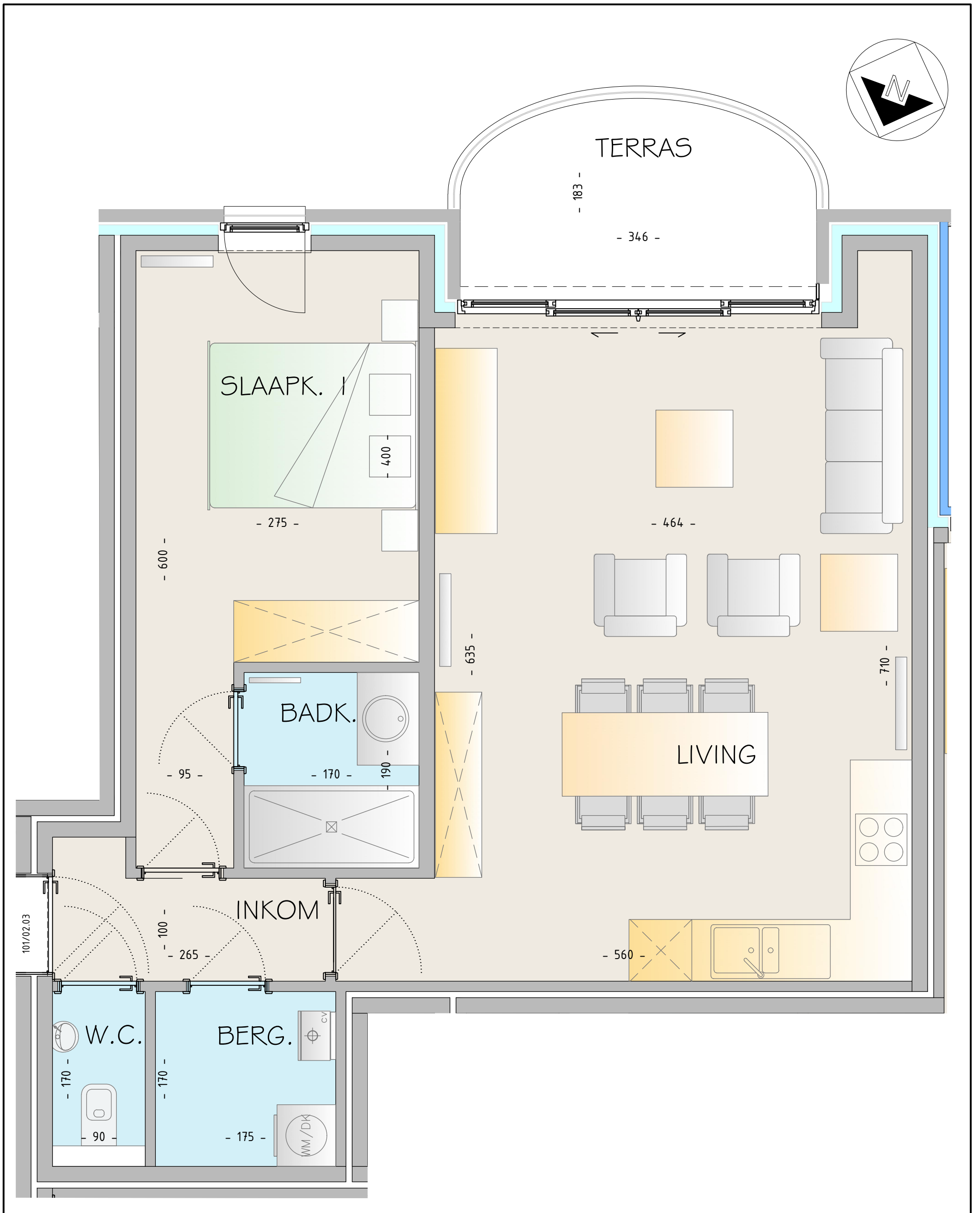
Appartement 101 / 02.03 Koninklijke Baan - B-8670 KOKSIJDE plandatum: 16/01/2019
